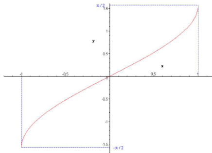
Figure – Graphes des fonctions sinus (à gauche) et arcsinus (à droite).
